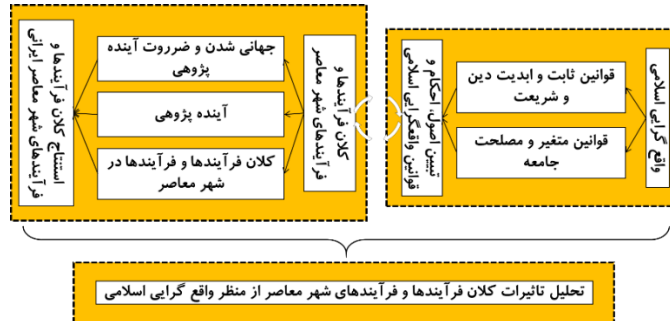
شکل ۴. فرآیند پژوهش
