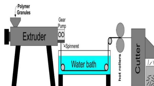
شکل ۴- دستگاه تولید الیاف
