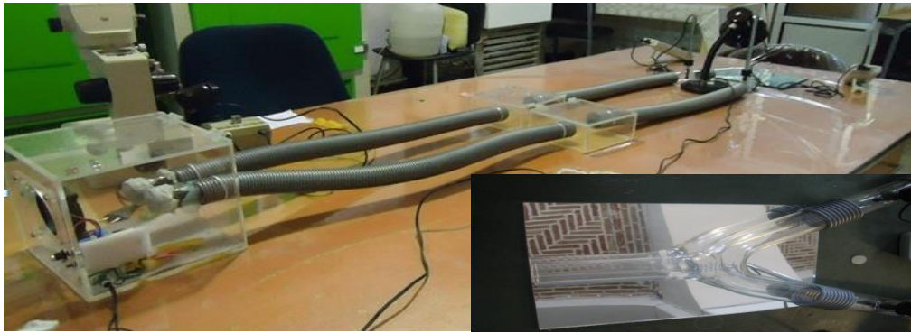
شکل ۱-لوله‌ی بوسنج
