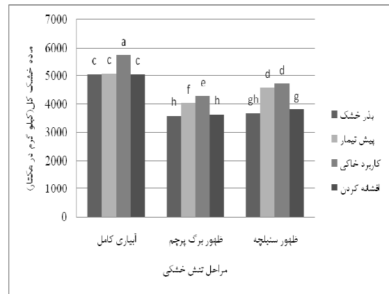
شکل ۱- اثر روش‌های کاربرد روی بر ماده خشک کل در مراحل مختلف تنش خشکی
