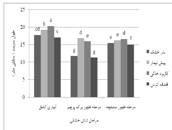
شکل ۳- اثر روش‌های کاربرد روی بر طول سربند در مراحل مختلف تنش خشکی
