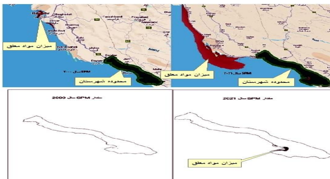
شکل ۷ برآورد میزان SPM سال ۲۰۰۰ (تصویر سمت چپ) و سال ۲۰۲۱ (تصویر سمت راست) منبع: سامانه ارث انجین
