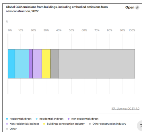
شکل ۲. انتشار جهانی CO2 از ساختمان‌ها، از جمله
